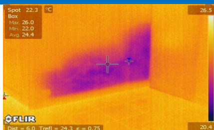
Humidité révélée par cartographie en infra-rouge
